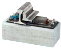
Innere Backenschienen- verspannung
